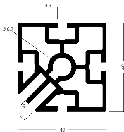
S 382 寸法 (mm)
