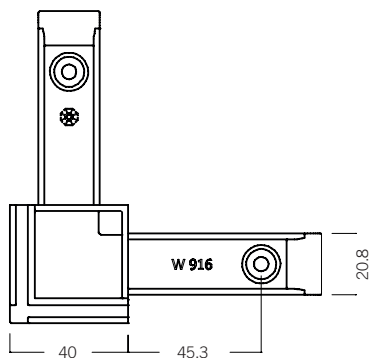
W 916 寸法 (mm)
