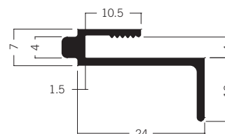
E 410 Door handle extrusion 0.50 kg
