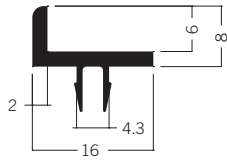
E 442 Supporting edge 0.40 kg
