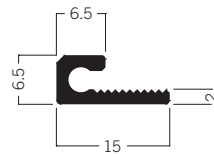
A 200* Edge protection 0.61 kg
