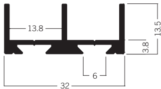
E 470/N* Sliding door extrusion 1.74 kg
