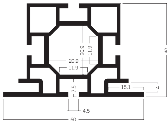
W 735R* Frame extrusion 60 mm universal (USA)
