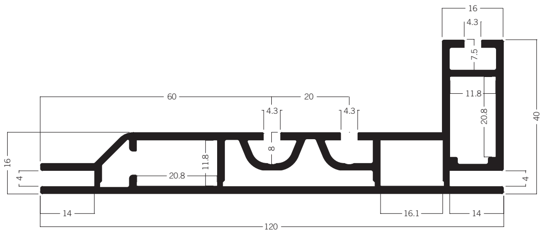
M 1915 Tension fabric extrusion für for light frame 120 mm 11.90 kg
