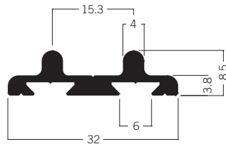
E 471/N* Sliding door extrusion 1.61 kg
